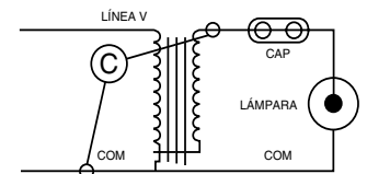
Entre cables común y del Capacitor
