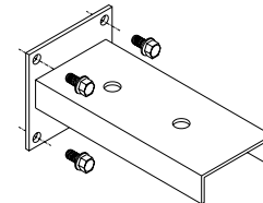
EWB - EXTENSIÓN DE MÉNSULA PARA PARED
