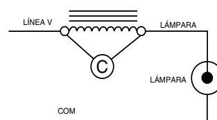
Entre cables común y del Capacitor
