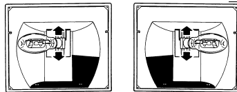
Ensamble del portalámparas de doble posición KL Distribución "D".
